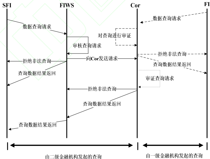
图例: SFI二级金融机构 FIWS拥有分支机构的一级金融机构 Cor协调节点 FI无分支机构的一级金融机构 ← SFI的查询路径 ← - - - FI的查询路径
